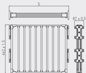
pełny wysuw / full extension / полное выдвижение
