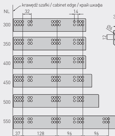
Rozstaw otworów montażowych Mounting dimensions Монтажные отверстия
